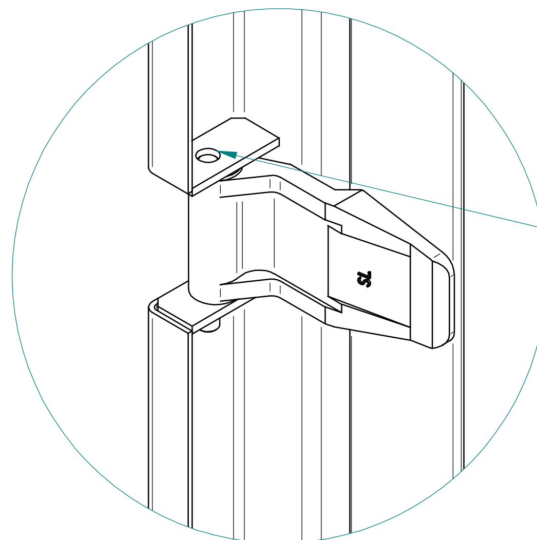
DETAIL B 1:2
